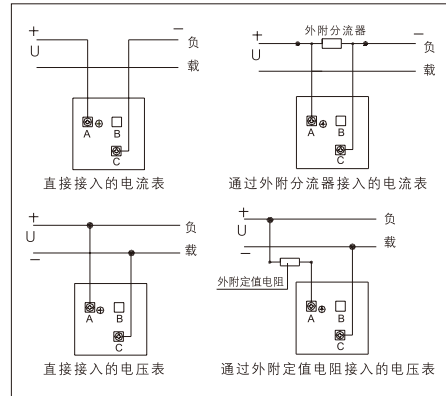
■ 96C-A、V, 72C-A、V接线图
