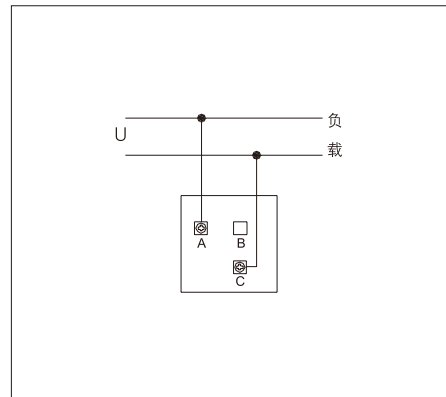
■ 96L-Hz, 72L-Hz接线图
