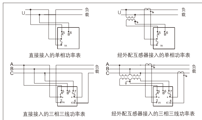
■ 72L-W、var接线图
