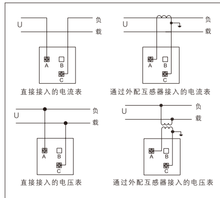
■ 96T-A、V, 72T-A、V接线图
