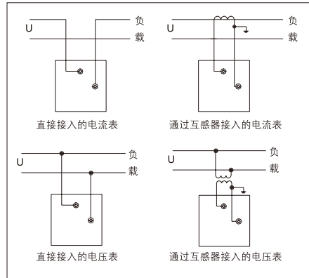
■ 99T1-A、V接线图
