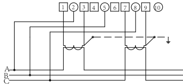
■ 三相三线电流互感器接入式接线图
