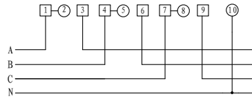
■ 三相四线直接接入式接线图
