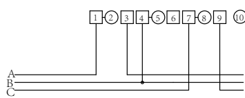
■ 三相三线直接接入式接线图
