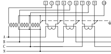
■ 三相四线电流、电压互感器接入式接线图
