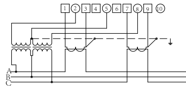
■ 三相三线电流、电压互感器接入式接线图
