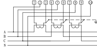
■ 三相四线电流互感器接入式接线图
